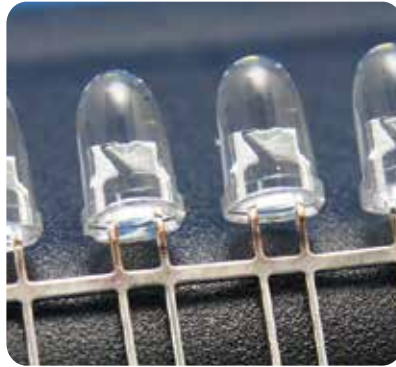
▲ 砲彈型 LED 外封裝膠
