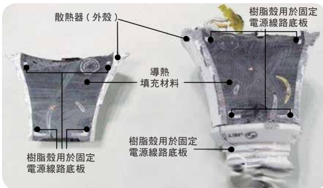
▲ 燈殼，螺旋後蓋與主體接著
