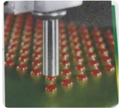
▲ SMT 貼片紅膠 - - 點膠用 (無鉛製程) 高速機
