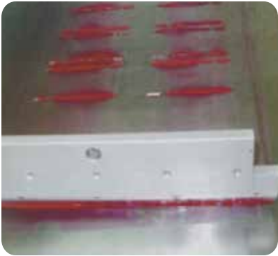
▲ SMT 貼片紅膠 - - 網印製程
